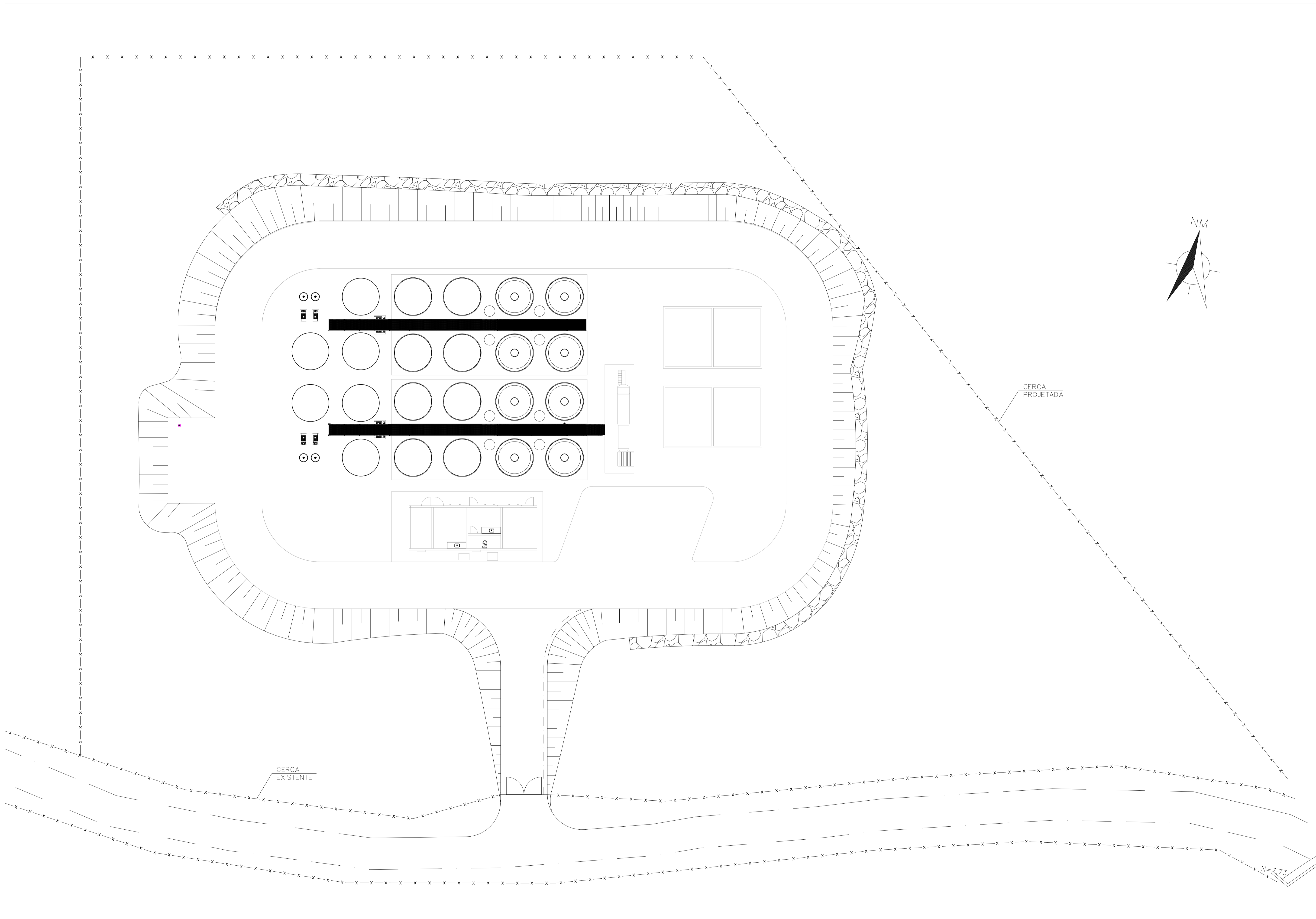
1 PLANTA GERAL 1: 150
